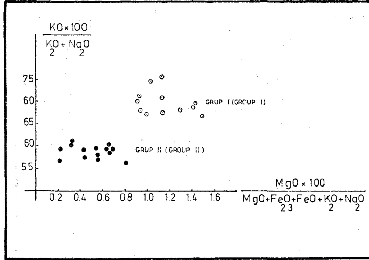
Şekil 2: Cumaovası asit volkanitlerine ait "Alkali İndeks-Katılaşma İndeksi" değişim diyagramı
